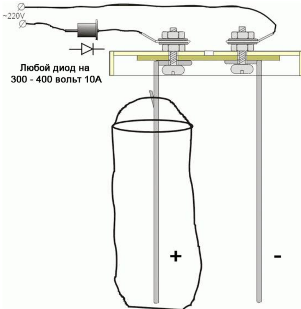
Схема прибора
